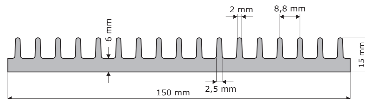
P3698 G=3,27 kg/m
