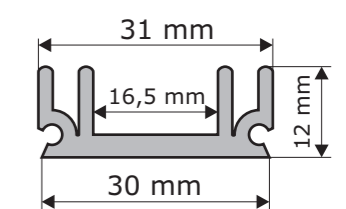
P22139 G=0,44 kg/m
