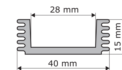
A4755 G=0,58 kg/m, F=2 cm 2
